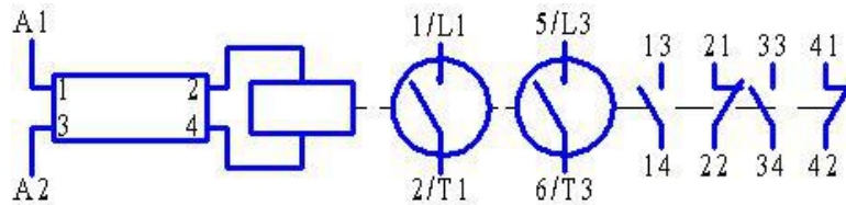
Рисунок Б.7 - KB2-400-2 с 2"З"+2"Р" вспомогательными контактами
