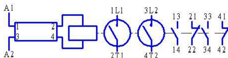
Рисунок Б.11 - KB2-630-2 с 2"З"+2"Р" вспомогательными контактами
