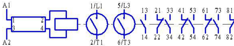
Рисунок Б.8 - KB2-400-2 с 4"З"+4"Р" вспомогательными контактами
