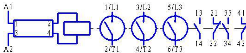
Рисунок Б.9 - KB2-400-3 с 2"З"+2"Р" вспомогательными контактами
