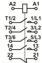
Рисунок 20. ПМЛ с доп.конт. 1з+1р
