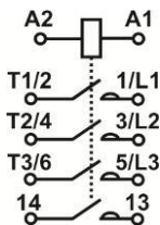
Рисунок 18. ПМЛ с доп.конт. 1з
